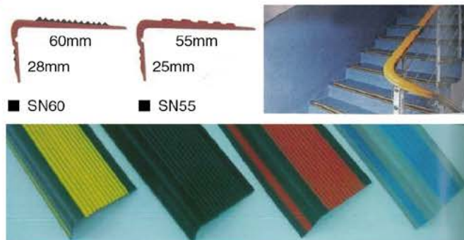
■ 防滑鋁合金吸咀 耐磨、防滑、表面PVC膠條
